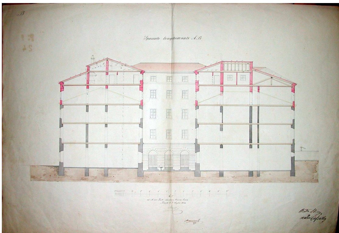
Progetto sopraelevazione – sezione longitudinale – 1856
