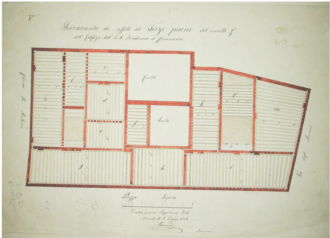
Travatura soffitti 3° piano – 1858
