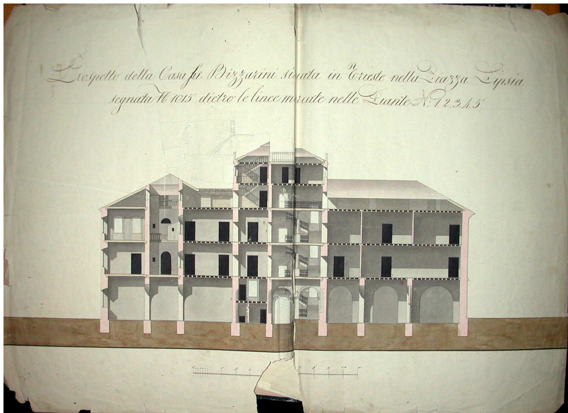
Sezione longitudinale
