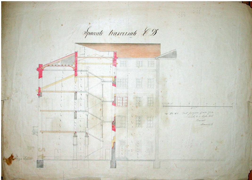
Progetto sopraelevazione – sezione trasversale – 1856
